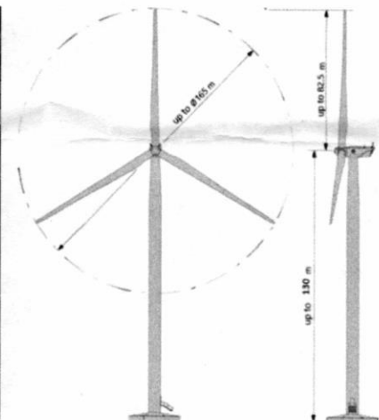
Характеристика на турбината
