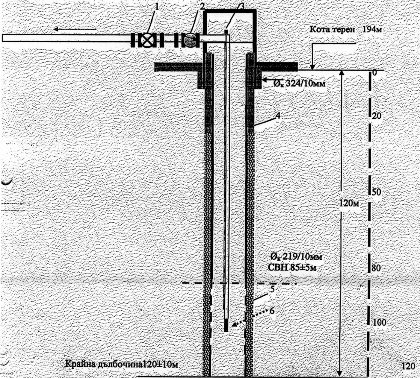
Фиг.8.Предвидено оборудване на ТК "ЗП Ивелина Годорова-Тригорци"-1-спирателен край, 2-водомер, 3-нивомер, 4-плътна колона, 5-филтрова колона, 6-помпа
