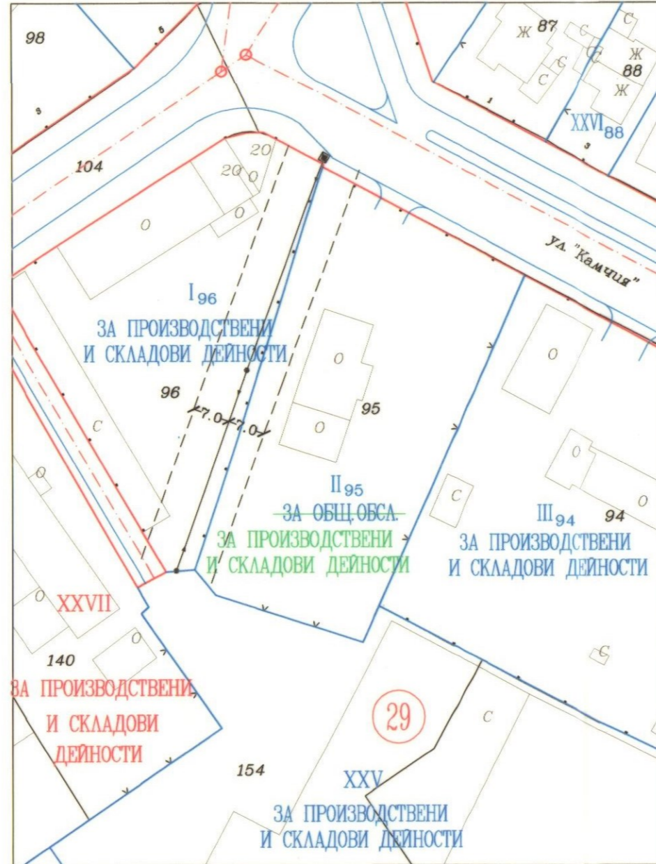
ИЗМЕНЕНИЕ НА ДЕЙСТВАЩИЯ ПУП – ПЛАН ЗА РЕГУЛАЦИЯ НА УПИ П-95, КВ. 29 ПО ПЛАНА НА ГР. БАЛЧИК, ОБЩ. БАЛЧИК
