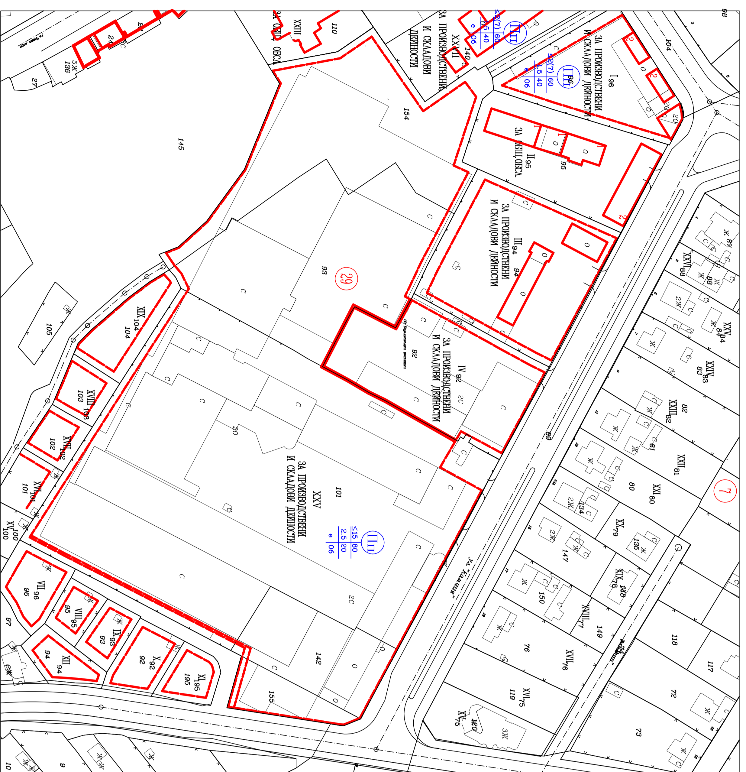
ИЗВАЛКА ОТ ДЕЙСТВИЕЩИ ПУП – ПЛАН ЗА ЗАСТРОЯВАНЕ НА УЛИЦИ П-95 И XXV, КВ. 29 ПО ПЛАНА НА ГР. БАЛЧИК, ОБЩ. БАЛЧИК
