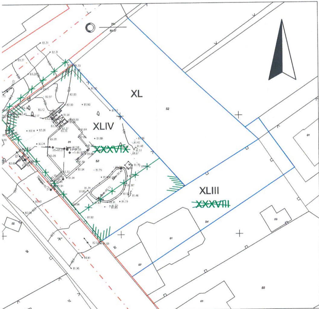
ПЛАН ЗА ИЗМЕНЕНИЕ НА РЕГУЛАЦИЯТА, М 1:500
