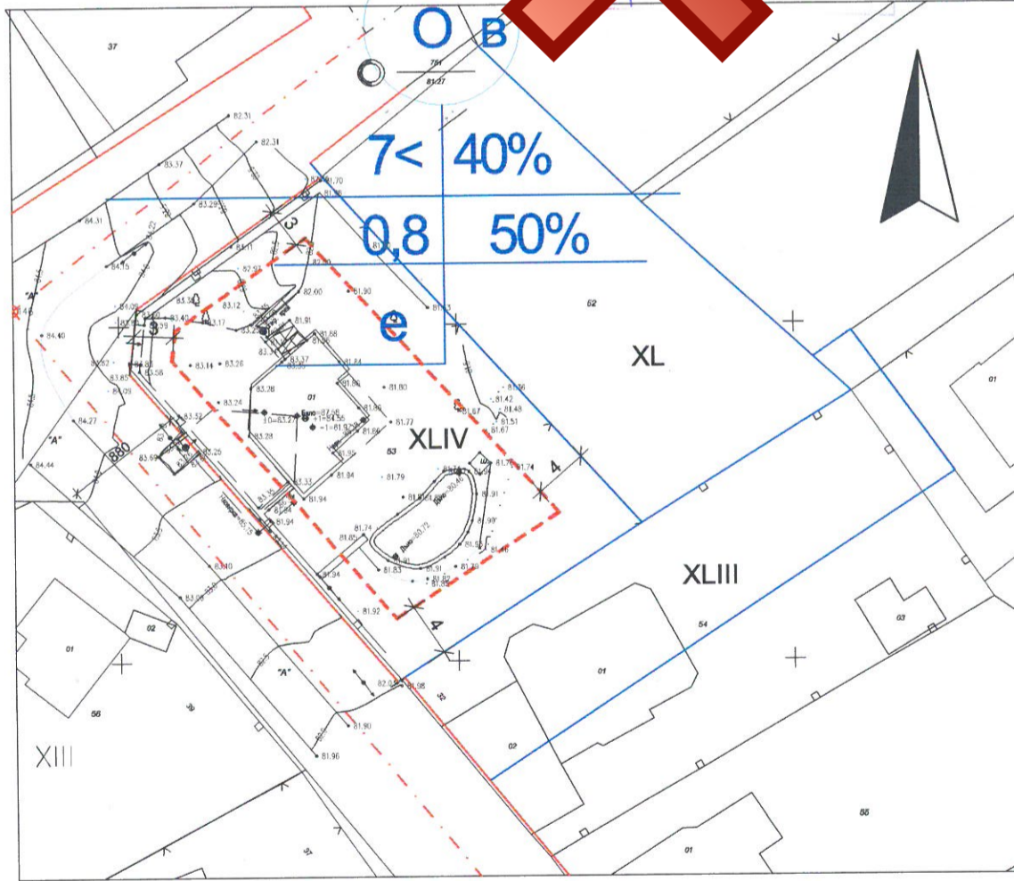
ПЛАН ЗА ЗАСТРОЯВАНЕ И РЕГУЛАЦИЯ, М 1:500
