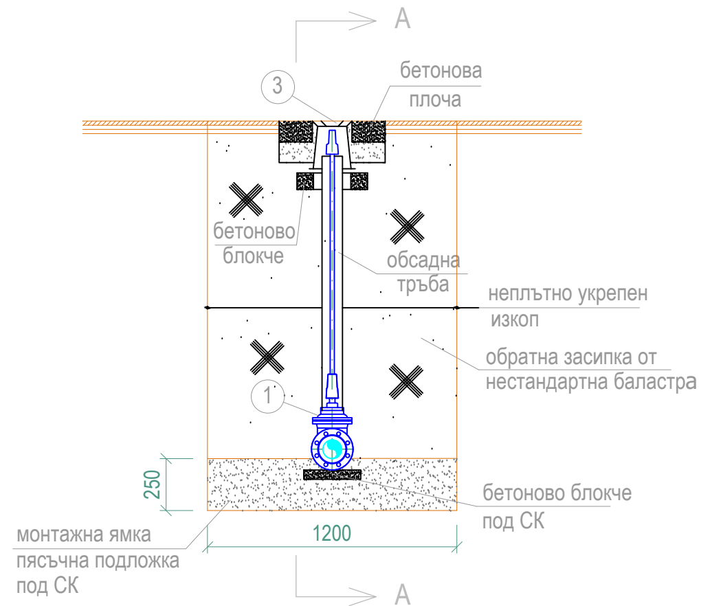
Вертикален разрез Б-Б
